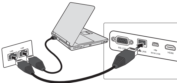
(连接示例)
